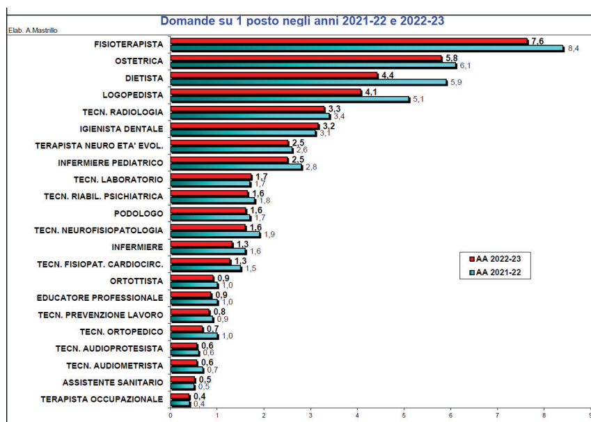
Figura 1 Rapporto tra D/P negli AA 2021-2 e 2022-3.
